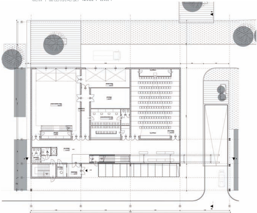
底层平面图(航站楼) NIVEL 0 LEVEL 0
