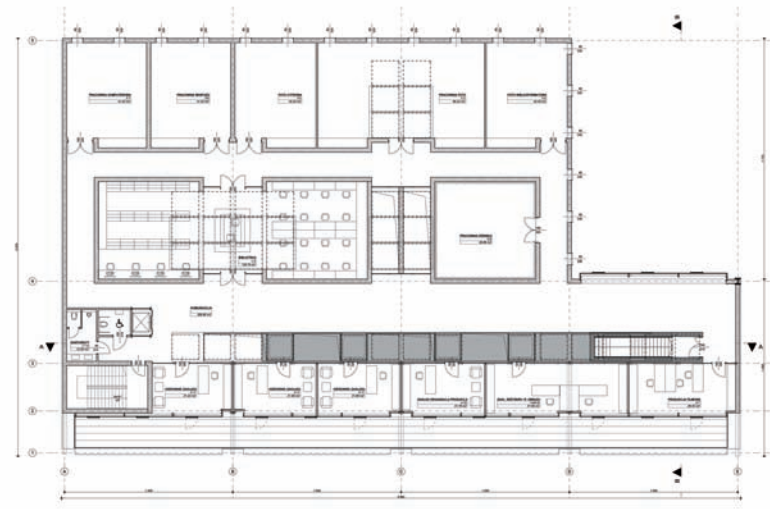
底层平面图(航站楼) NIVEL 2 LEVEL 2
