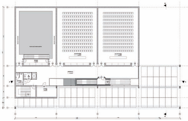
底层平面图(航站楼) NIVEL 1 LEVEL 1
